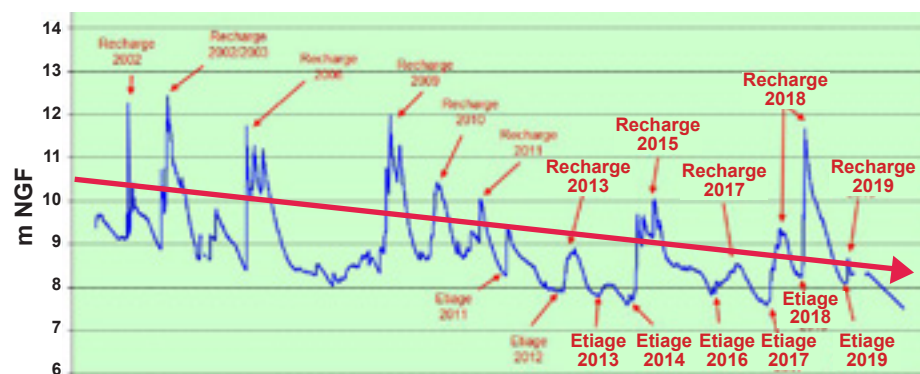
Evolution piézométrique de la nappe de la Vistrenque, forage Mas Faget, Codognan - EPTB Vistre-Vistrenque
