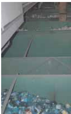
Triage des métaux grâce à un aimant et les bacs de selection.
