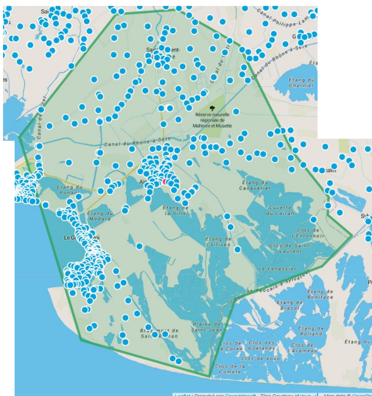
FIGURE 40 : POSTES DE TRANSFORMATION HTA/BT ET POSTE SOURCE (HTB/HTA) DU RESEAU ELECTRIQUE (DONNEES : ENEDIS)
